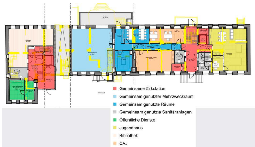
Skizze Erdgeschoss
